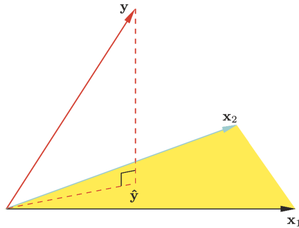
Figura 1.8: Ilustración de la poroyección de y en x_1 y x_2 y el significado del error e , retomado de Hastie, Tibshirani y Friedman (2009, pp. 46) [HTF17]
