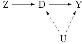
Figura 1.3: Ejemplo 4 de un DAG, estimador basado en variables instrumentales
